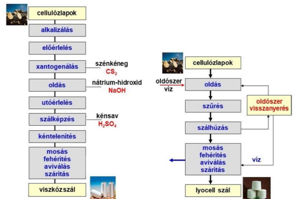
A viszkóz- és a lyocell szálgártási technológiáinak összehasonlítása
